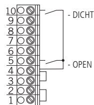
Sleutelschakelaar
