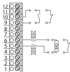
Ingang 1 (9 + 10) Sluitkantbeveiliging 8,2 k \Omega / DW (5+6)
