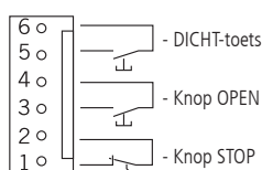
Klepknoppen KDT
