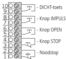
Bedieningsapparaten
